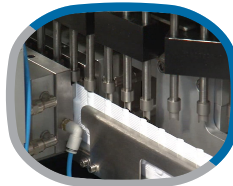
• Thermoforming station for plastic films • Station formage des matériaux plastiques • Kunststoffsformungsstation
